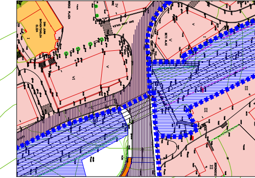
beheko planoa_plano inferior
